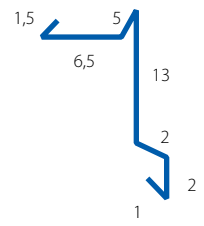
Záveterná lišta- škridla Obrobka 35K
