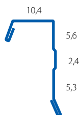
Záveterná lišta profilovaná Obrobka 121
