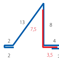
Snehová zábrana WSPORNIK-SK | SNIEG-SK
