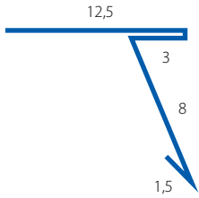
Štartovacia lišta - Klik Panel Obrobka 4
