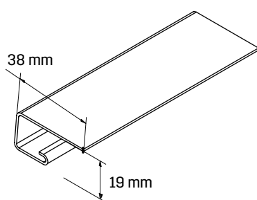
Montážna lišta J
