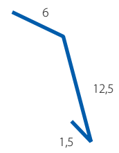
Nadžľabový pás Obrobka 7
