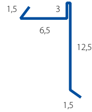
Záveterná lišta dolná Obrobka 3
