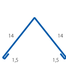
Hrebenáč hladký Obrobka 205K
