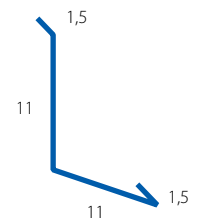
Napojenie na stenu dolné Obrobka 12
