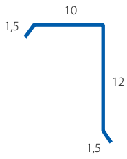
Záveterná lišta Obrobka 1
