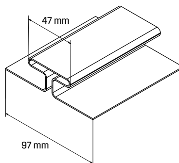
Montážna lišta H
