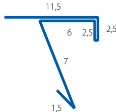
Štartovacia lišta - modul Obrobka 5
