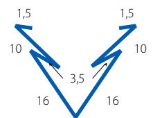
Úžľabie Obrobka 185K
