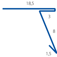
Štartovacia lišta - Klik Panel Obrobka 45K
